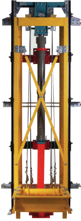
HİDROLİK KARKAS VE PİSTON
