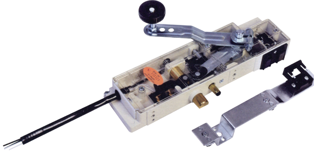
ÇİFT DİLLİ ÇİFT EMNİYETLİ ASANSÖR KAT KAPI KİLİDİ
