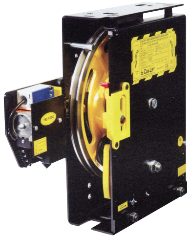
ÇİFT YÖNLÜ AŞIRI HIZ REGÜLATÖRÜ
